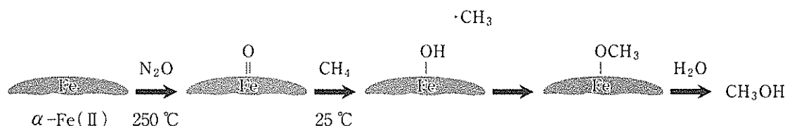
図 \alpha -Fe(II) 上で起きるメタンのメタノールへの変換（概略図）
