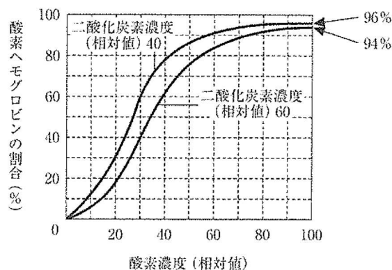
図1. 酸素解離曲線
