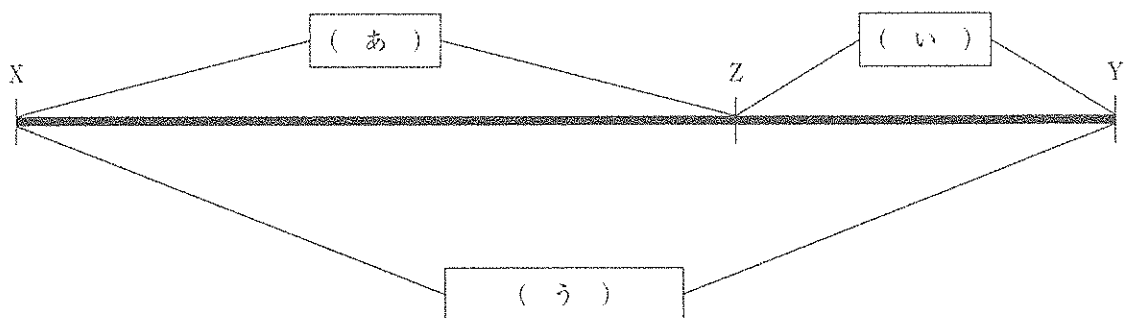
図1. 同一染色体上における遺伝子 X, Y, Z の位置
