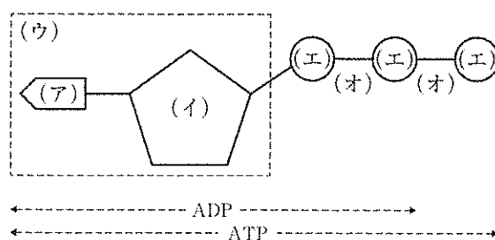
図1. ADPとATPの構造
