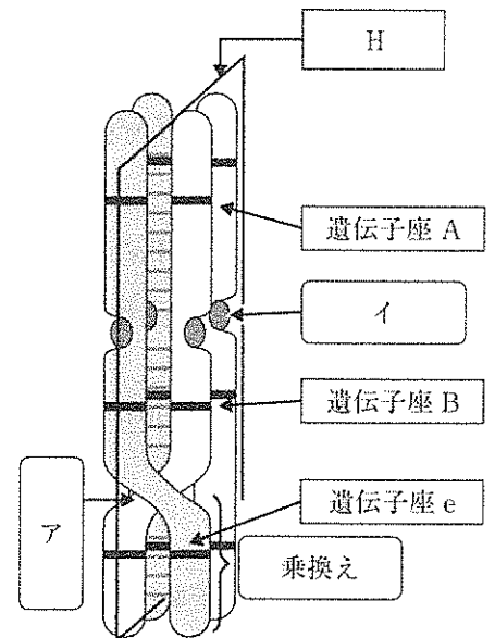
図2. 染色体の乗換え
