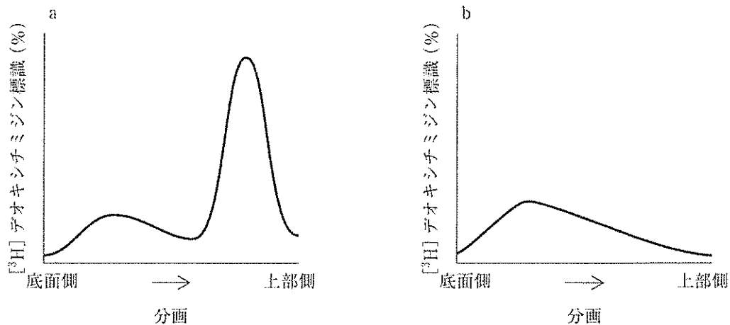
図3. 仮説モデルより予想される実験結果のパターン
