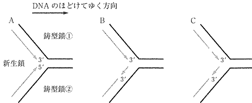
図2. DNA複製領域の構造と反応の仮説モデル
