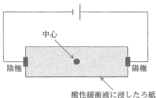
図1 グリシンの電気泳動
