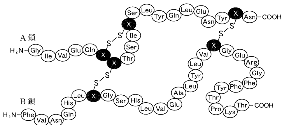
図2 ヒトのインスリンの一次構造
