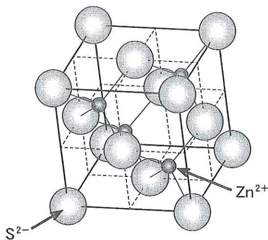
図 1 硫化亜鉛の立方体形の単位格子
