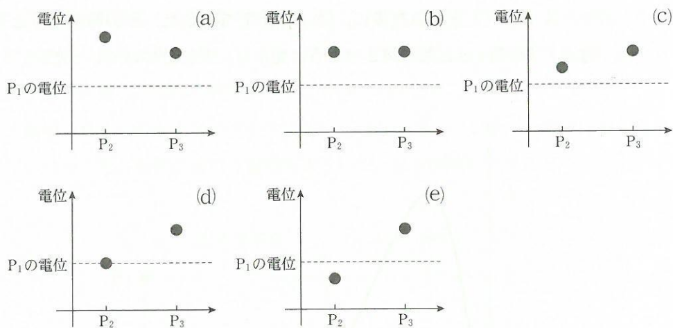
図3 空欄 オ の選択肢。横軸は回路上の点の位置を示す。
