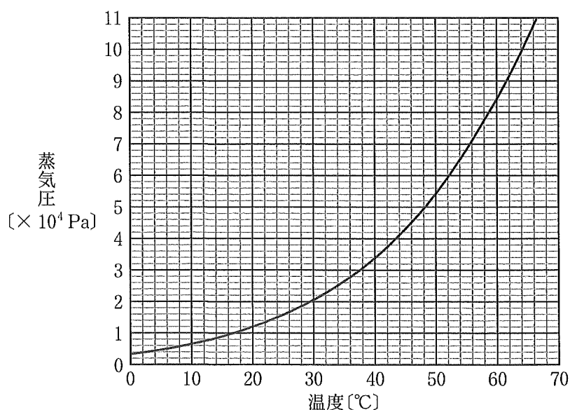
図 2 メタノールの蒸気圧曲線
