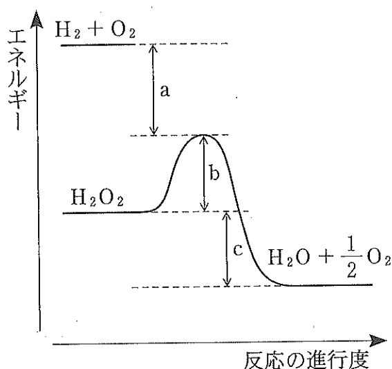
図1 過酸化水素の分解反応におけるエネルギー変化。単体の \text{H}_2 と \text{O}_2 の混合物の状態もあわせて示す
