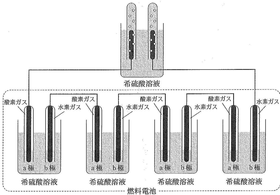
図1. グローブ卿の燃料電池
