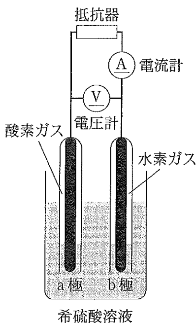
図 2. 実験用回路
