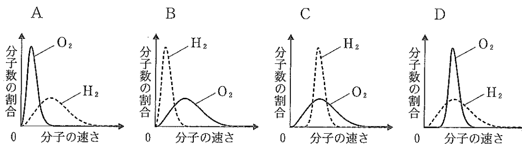
図 気体分子の速度分布
