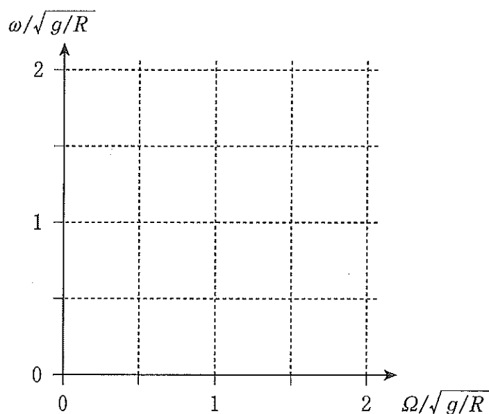
図 2 リングの回転角速度 \Omega と、物体の微小振動の角振動数 \omega の関係
