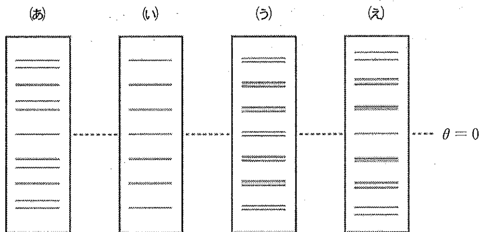
図2 スクリーンと明線のパターン。各図の四角が図1におけるスクリーンを表し、その中の線が明線を表す。各図の縦方向の中心(図中の点線)が図1における \theta = 0 の位置に対応する。明線の明るさや色は図には反映されていない。
