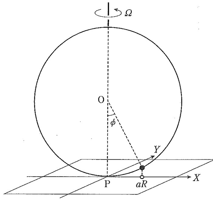
図3 物体の水平面内での位置を示す座標( X , Y )
