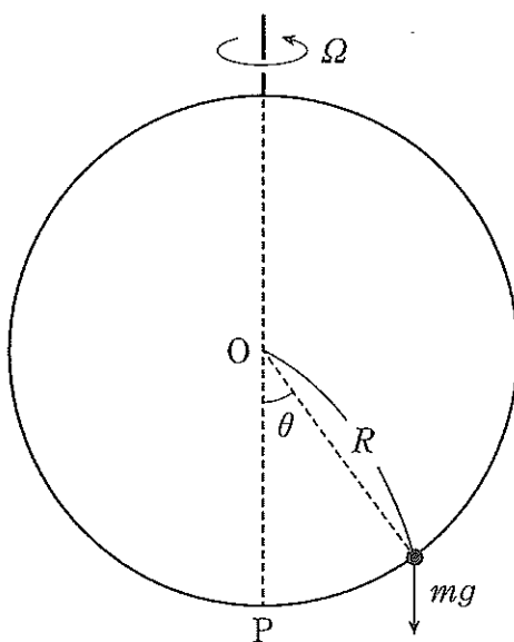
図 1 回転するリング上を動く物体
