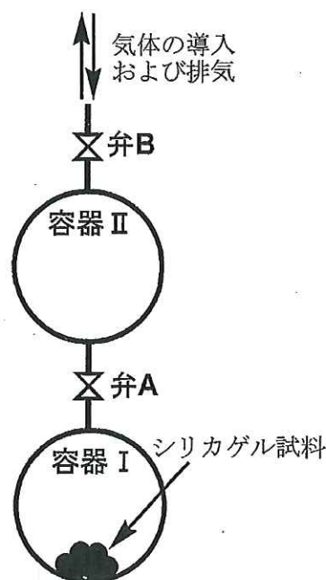
図2 実験装置
