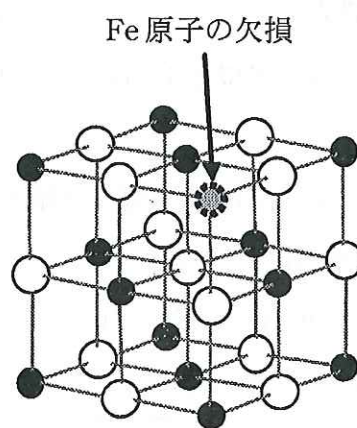
図 2 Fe 原子の欠損の一例
