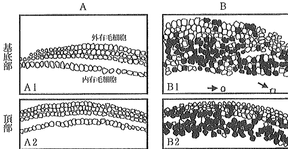
図3 基底膜上の内有毛細胞と外有毛細胞の分布（有毛細胞と判定されたもののみを示してある。支持細胞は多数あるがこの図には示していない。） A：プラスミドを注入していない個体。B：プラスミドを注入した個体（黒く塗りつぶしたものは緑色蛍光を発している有毛細胞）。B1での矢印は本来、有毛細胞が現れないところに観察された有毛細胞を示す。A1, B1：蝸牛の基底部分での分布、A2, B2：蝸牛の頂部での分布
