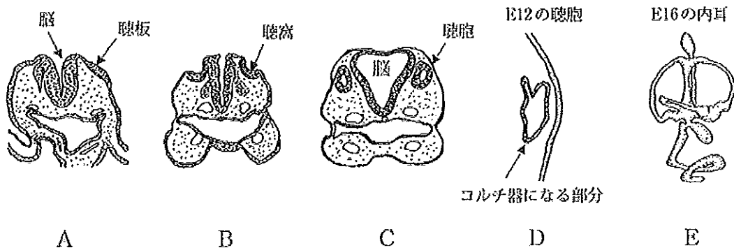
図 2 ほ乳類の蝸牛の発生過程
