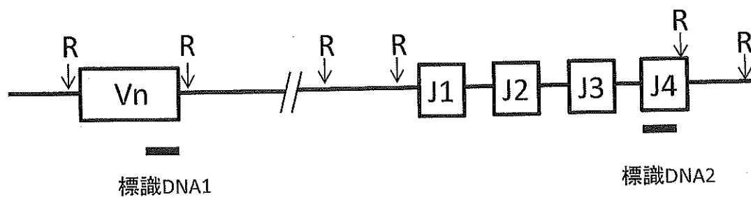
図2 抗体遺伝子の構造(再構成に関係する一部分のみを示す)
