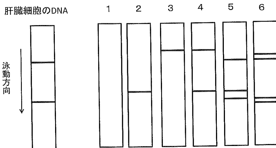
図3 抗体遺伝子領域の電気泳動のパターン
